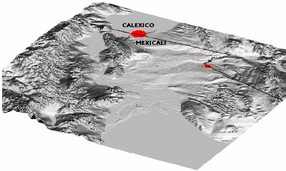
Figura 3.2. Topografía de la región
