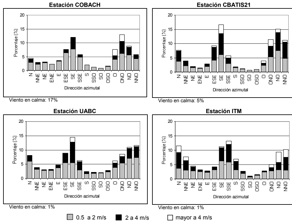
Figura 4.4. Dirección y velocidad del viento en Mexicali, 1997 (Porcentaje de ocurrencia por dirección y velocidad)
