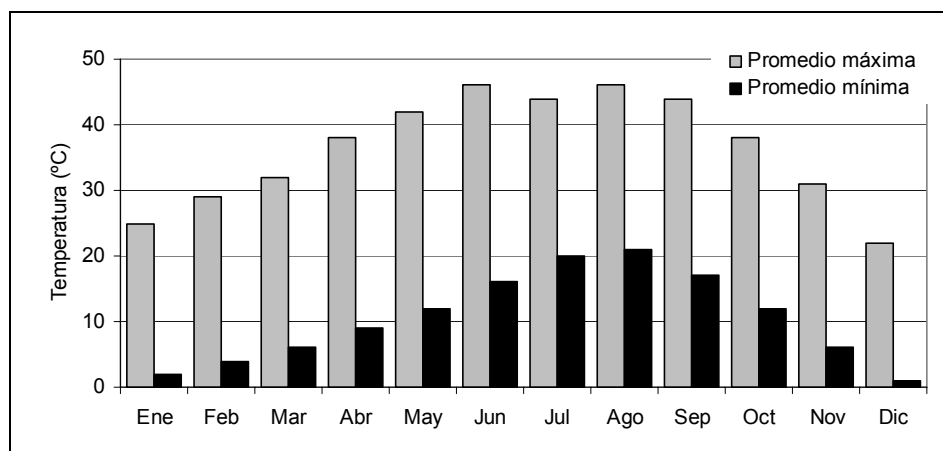
Figura 4.5. Promedios de las temperaturas máximas y mínimas mensuales en Mexicali, 1981-1997
