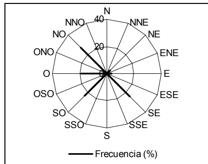
Figura 4.1. Rosa de viento dominante en Mexicali, 1996 (porcentaje y dirección)
