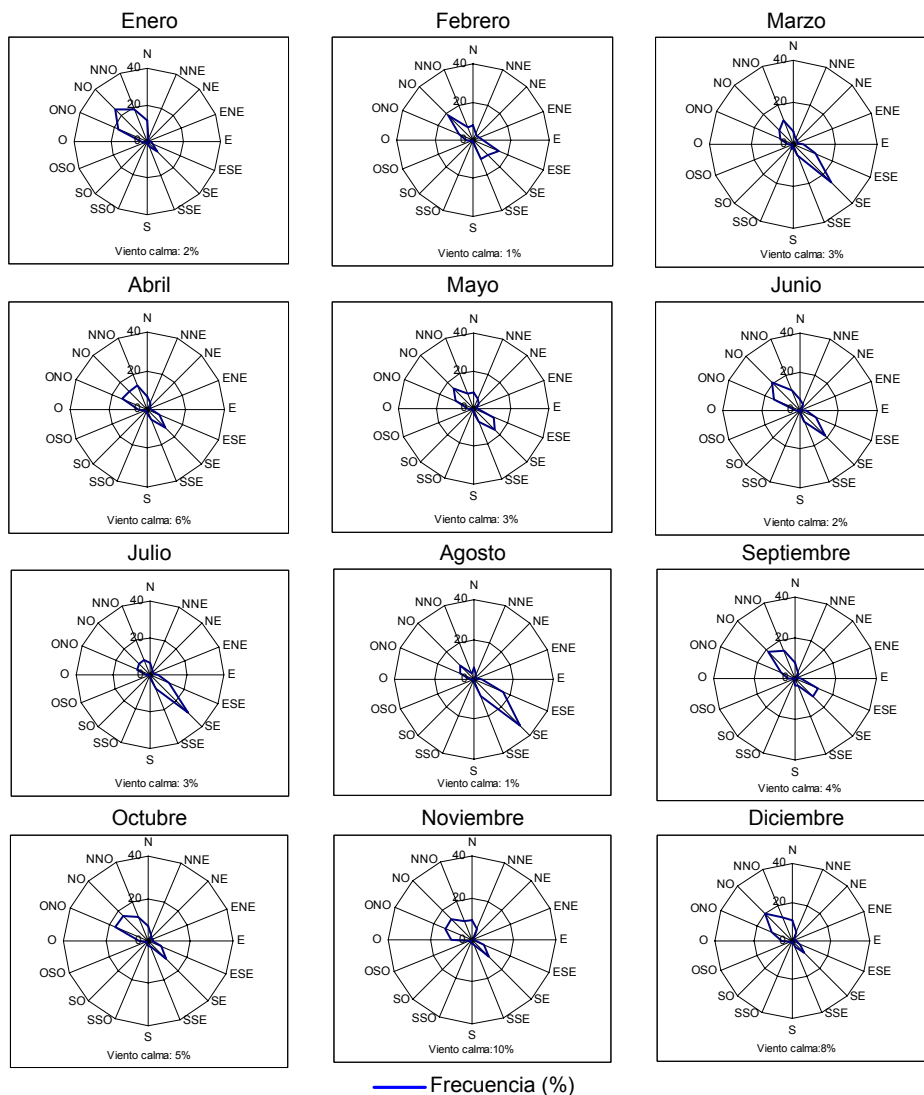
Figura 4.3 Rosa de viento por mes en Mexicali, 1997
