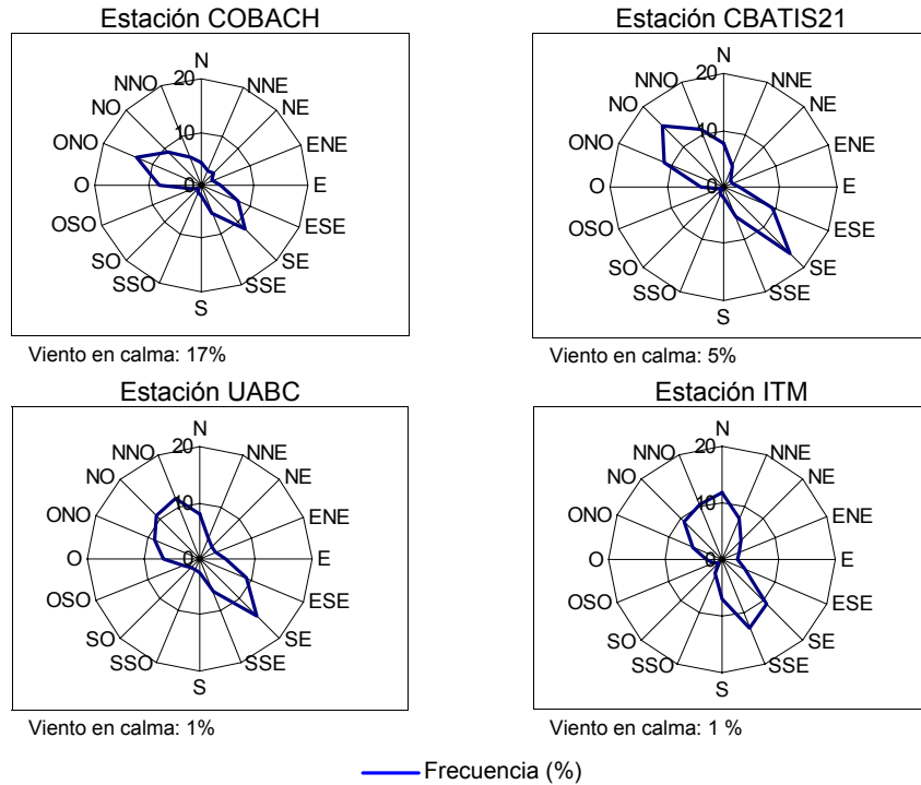
Figura. 4.2. Rosa de viento en las estaciones de monitoreo de Mexicali, 1997 (porcentaje y dirección)
