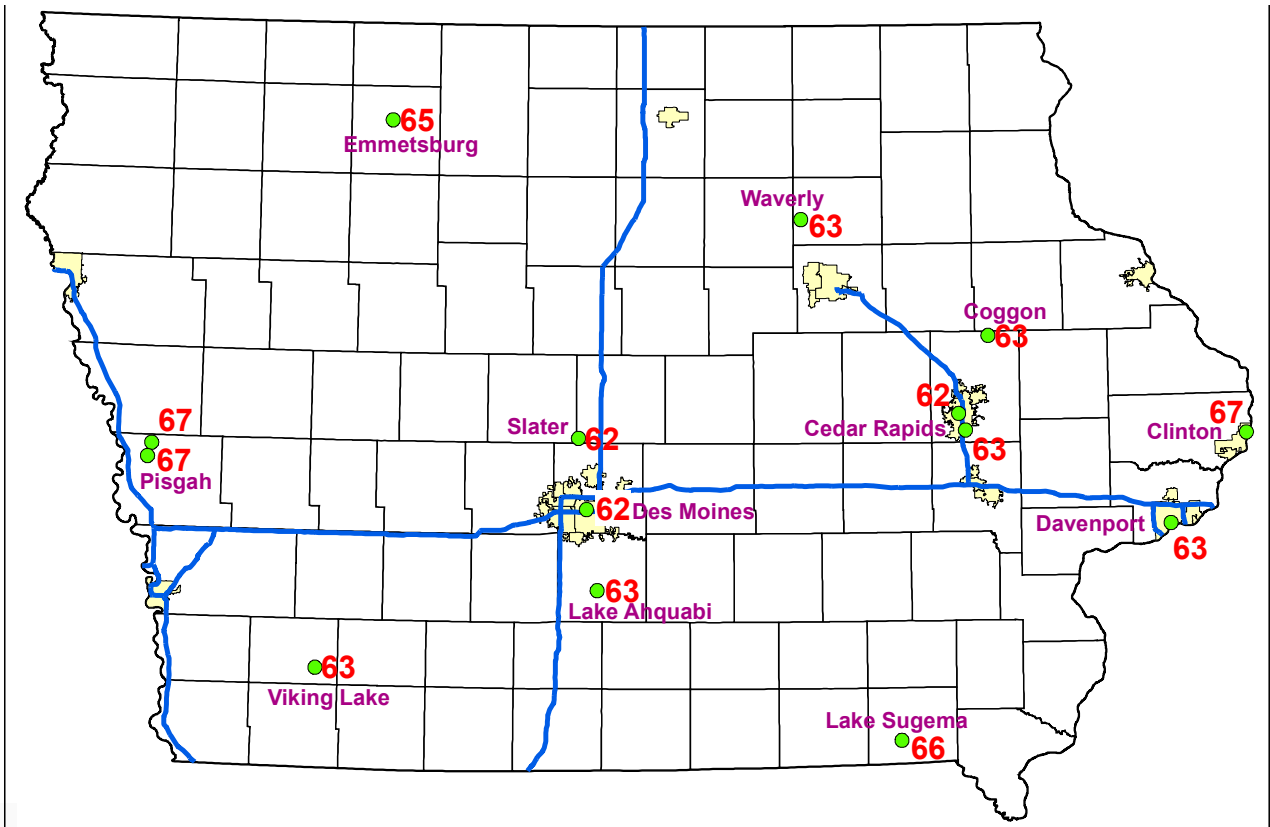
2012-2014 Ozone Design Values (ppb)
