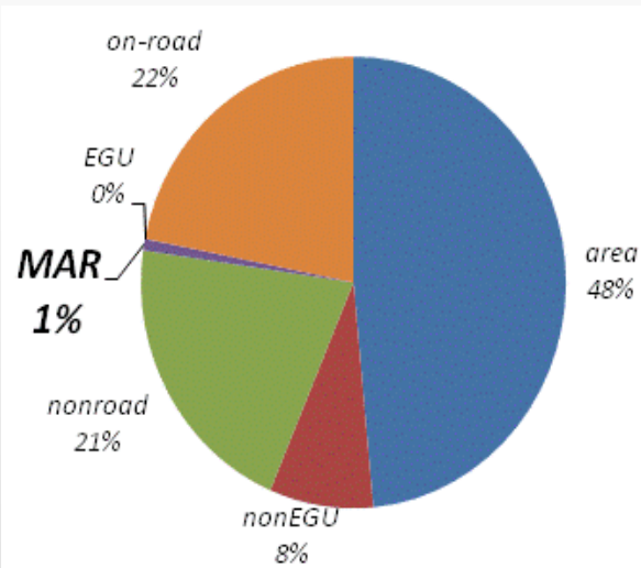
VOC
