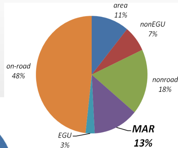
NO x
